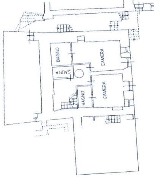
PIANO PRIMO SEMINTERRATO H = 2,30 m
